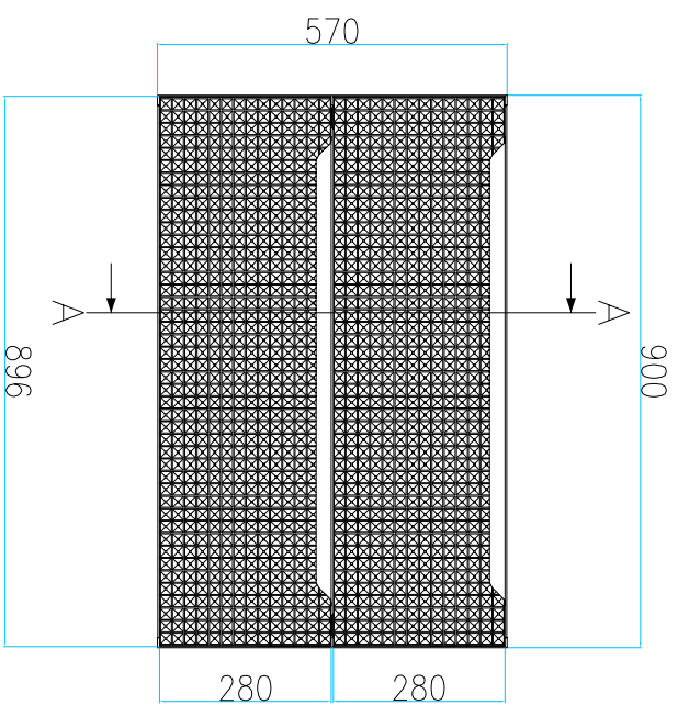
Widok 1
