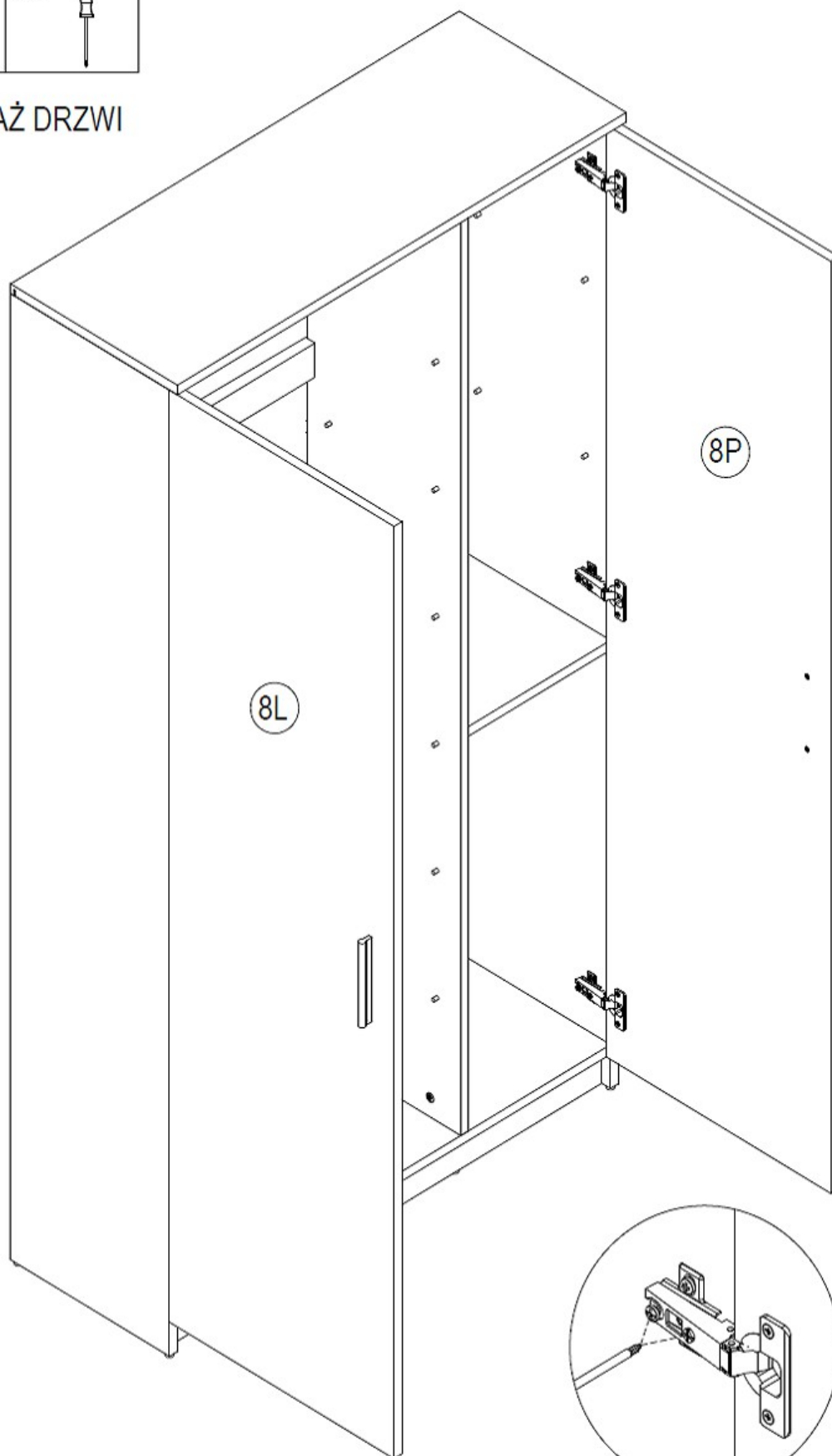
łączenie i regulacja zawiasu
